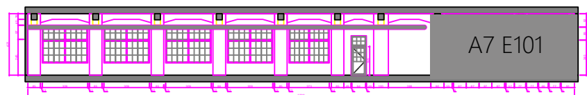
IE-A-01 立面圖(一)
